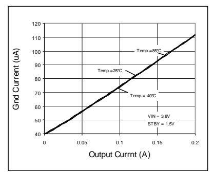
Fig. 97 IOOUT - IIGND
