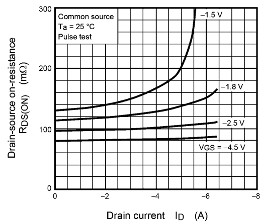
Fig. 7.4 R_{DS(ON)} - I_D
