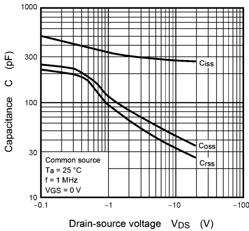
Fig. 7.9 C - V_{DS}
