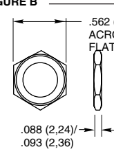
Hex Nut
