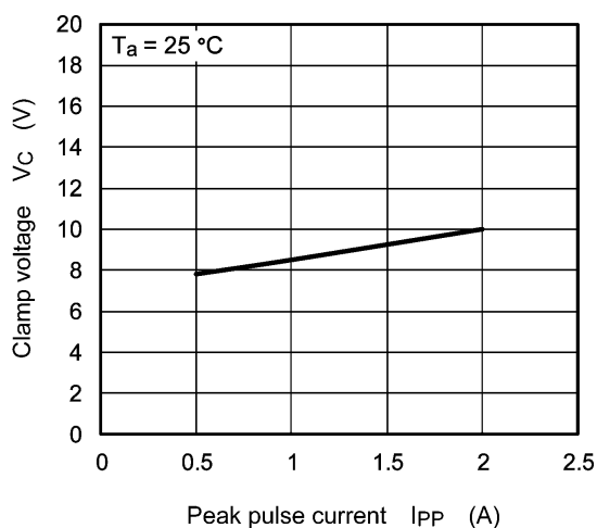
Fig. 6.3.1 V_C - I_{PP}
