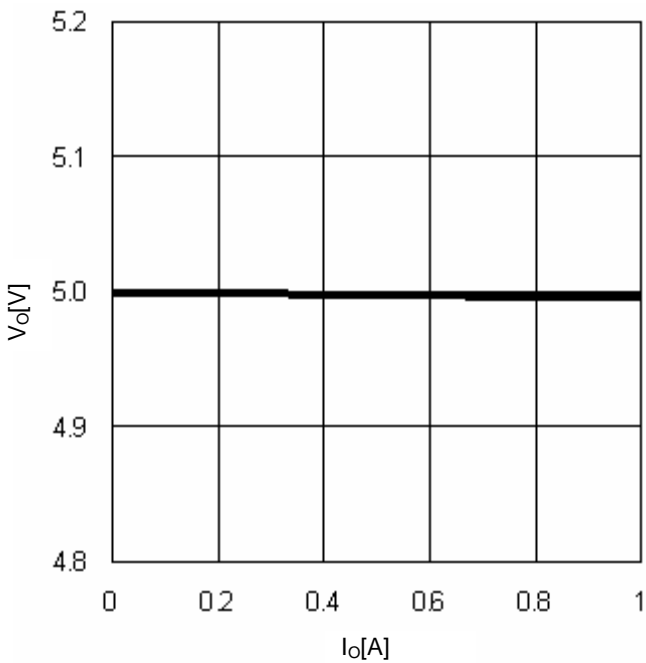
Fig.12 I_O - V_O
