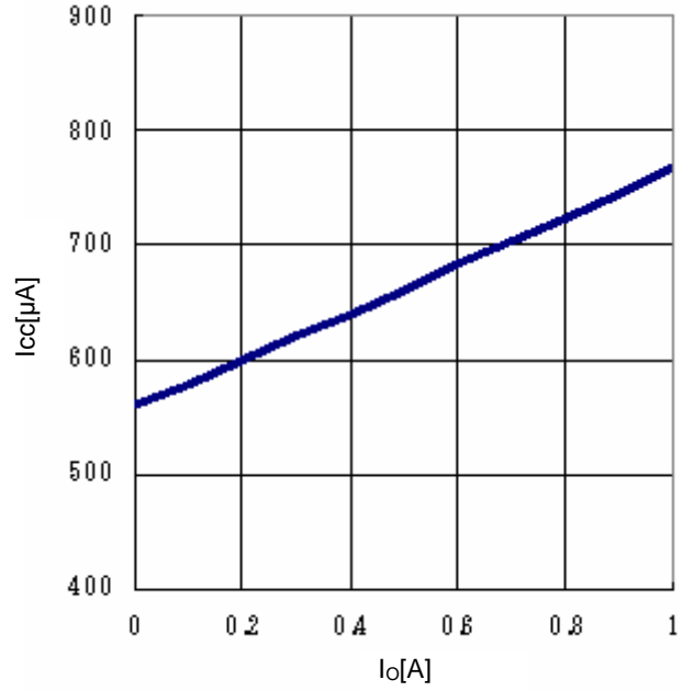
Fig.19 I_o - I_{cc}
